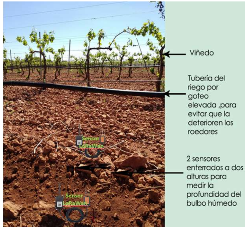
Sensores en el control del riego de viñedos
